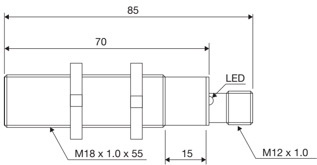
Fig. 8 Plug CA18EAF...M1IO
