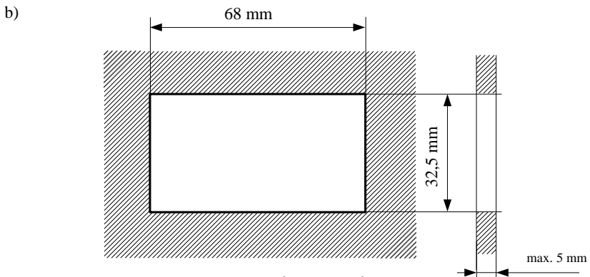
Hình 4.1. Kích thước lỗ lắp: a) khuyến nghị b) cho phép
