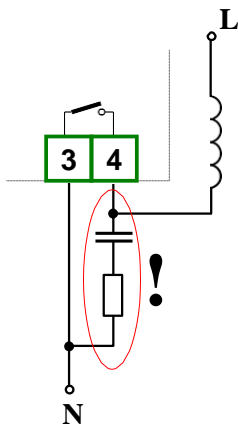
Hình 4.8. Kết nối mạch triệt tiêu:
