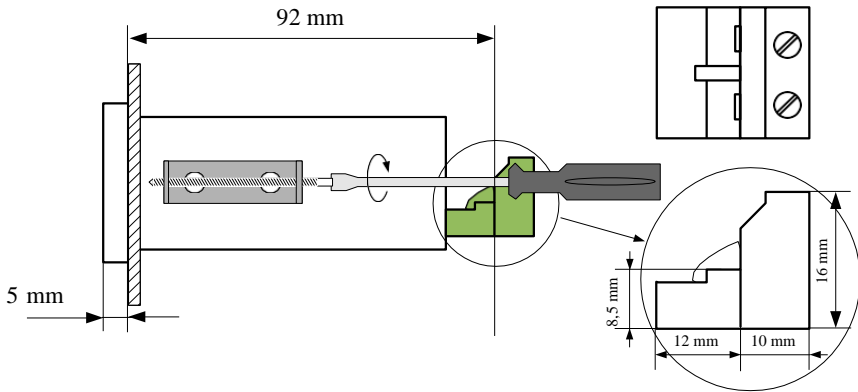
Hình 4.2. Lắp đặt giá đỡ và kích thước của đầu nổi.
