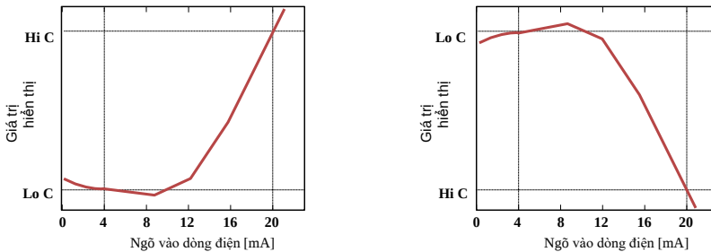
Figure. 10.2 Đặc tính thường („Lo C” < ”Hi C”) và nghịch đảo („Lo C” > ”Hi C)
