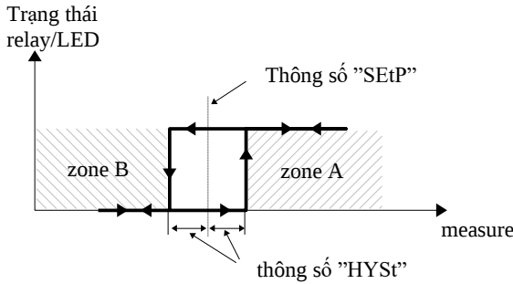
Figure 6.5. Một ngưỡng điều khiển của các ngõ ra rơ le / đèn LED
