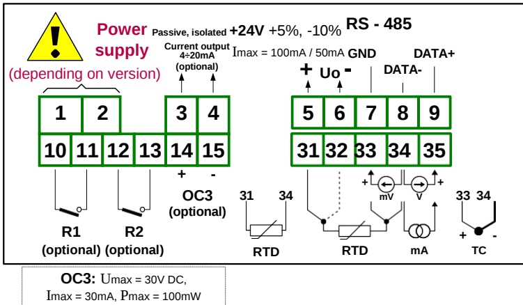
Figure 4.11. Thiết bị chân kết nối (Ngõ ra hai rơ le, một loại OC và một dòng điện passive)
