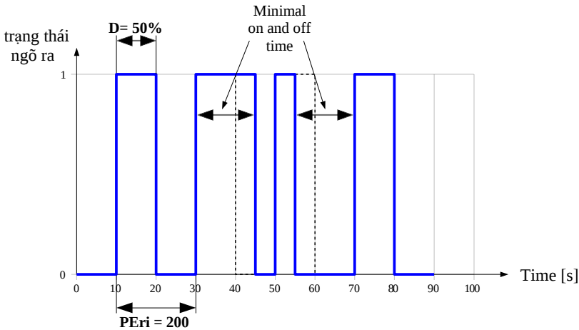
Figure 6.10. Tiến trình của tín hiệu ngõ ra PWM loại OC trong chế độ PULS
