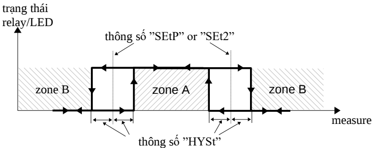
Figure 6.6. Hai ngưỡng của ngõ ra rơ le / đèn LED
