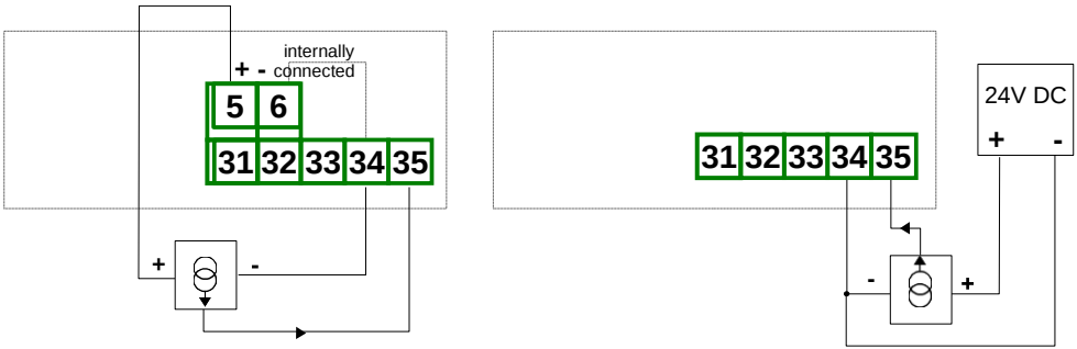
Figure 4.14. Kết nối bộ chuyển đổi dòng điện 3 dây
