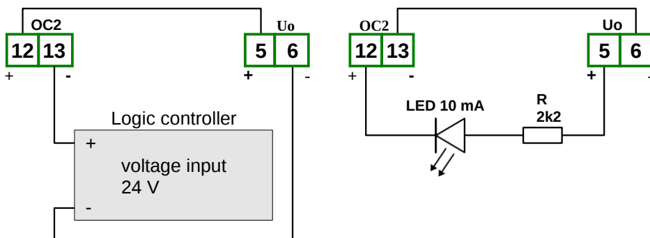
Figure 4.19. kết nối ngõ ra kiểu OC (chỉ dành cho thiết bị có ngõ ra kiểu OC)
