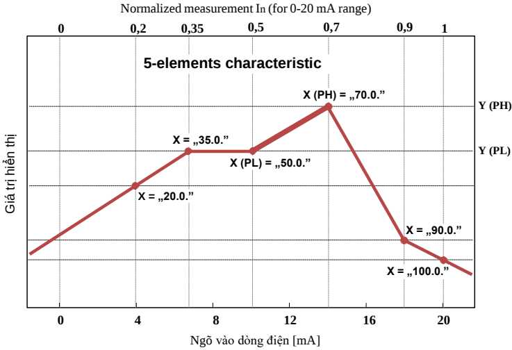
Figure. 10.4 Ví dụ về đặc tính do người dùng xác định
