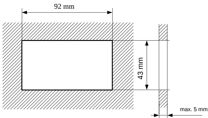
Figure 4.1. Kích thước lỗ lắp được đề xuất
