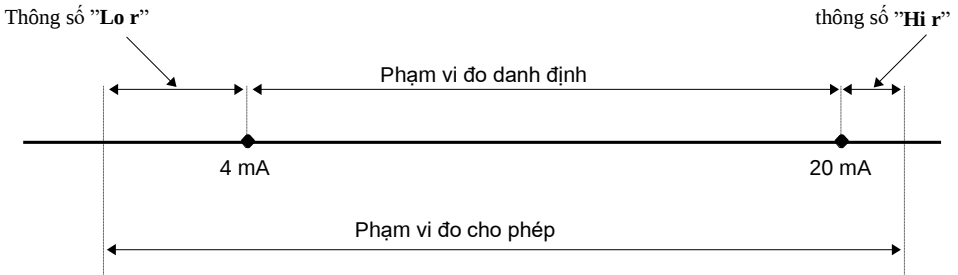
Figure 6.1. Phạm vi đo lường trong chế độ 4 \div 20\text{mA}
