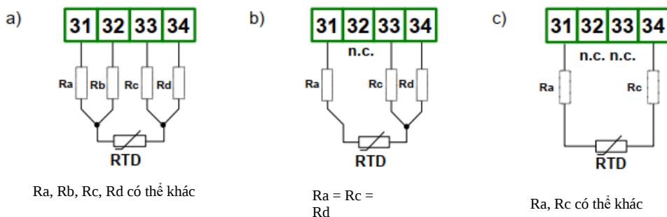
Figure 4.16. Kết nối các cảm biến RTD: a) Mạch 4-dây; b) Mạch 3-dây; c) Mạch 2-dây
