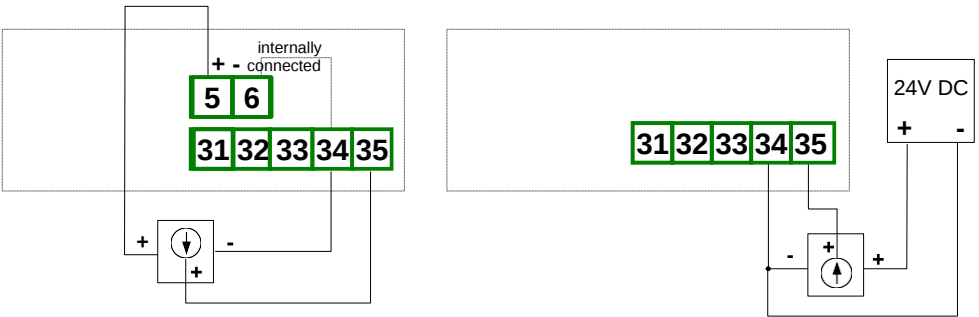
Figure 4.15. Kết nối đầu dò điện áp
