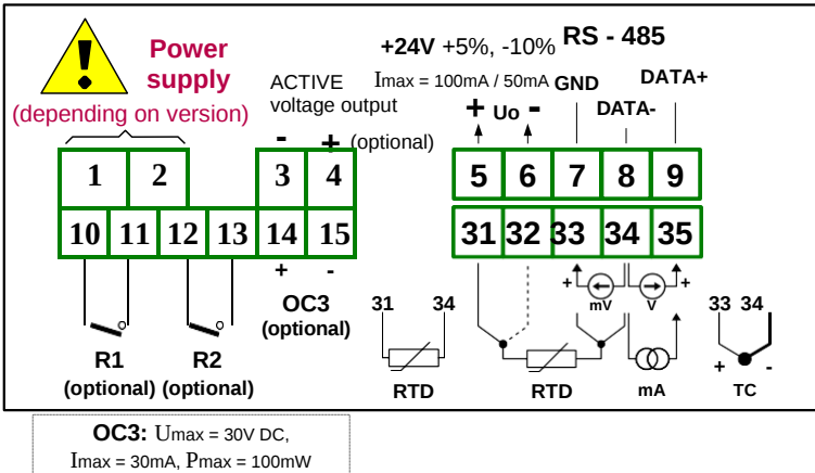
Figure 4.12. Thiết bị chân kết nối (Ngõ ra hai rơ le, một loại OC và một điện áp active)
