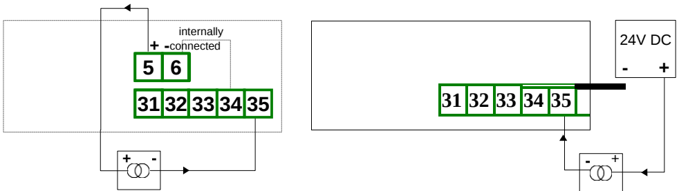
Figure 4.13. Kết nối bộ chuyển đổi dòng điện 2 dây
