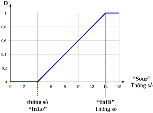
Figure 6.9. Đặc điểm của tín hiệu ngõ vào - ngõ ra ở chế độ "PULS" cho các tham số: "InLo" = 4, "InHi" = 14
