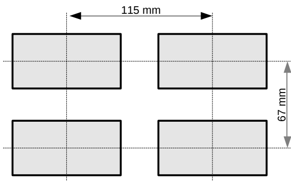
Figure 4.3. Lắp đặt giá đỡ và kích thước của đầu nối.
