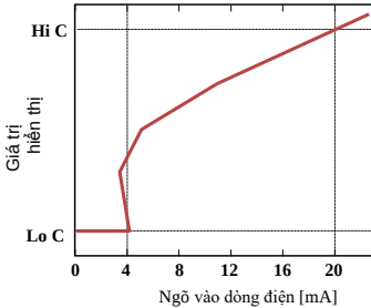
Figure. 10.3 Đặc tính thường („Lo C” < ”Hi C”) và nghịch đảo („Lo C” > ”Hi C)
