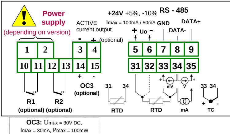
Figure 4.10. Thiết bị chân kết nối (Ngõ ra hai rơ le, một loại OC và một dòng điện active)
