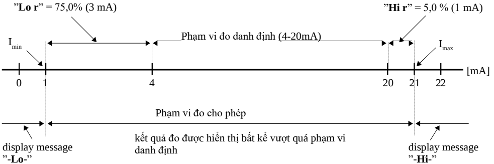
Figure 7.3 Ví dụ về định nghĩa phạm vi cho phép của tín hiệu ngõ vào - thông số "Lo r" và "Hi r" (chế độ "4-20")
