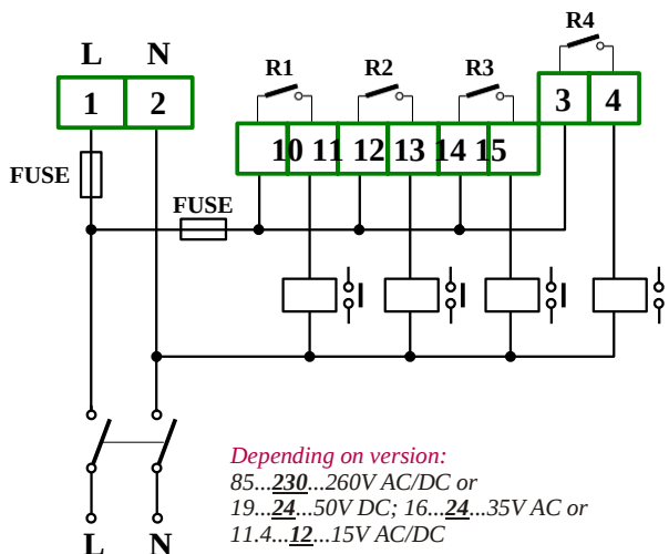
Figure 4.17. Kết nối nguồn điện và rơ le
