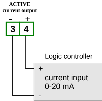
Figure 4.20. Kết nối ngõ ra dòng điện active (chỉ dành cho thiết bị có ngõ ra dòng điện active)
