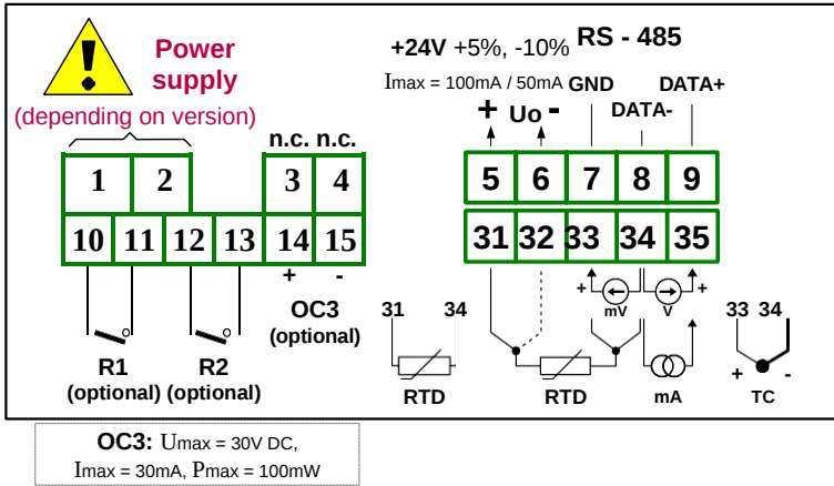
Figure 4.9. thiết bị chân kết nối (hai ngõ rơ le và một ngõ ra OC)
