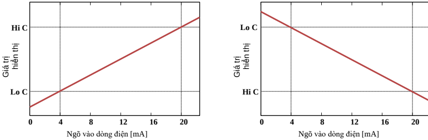
Figure. 10.1 Đặc tính thường („Lo C” < ”Hi C”) và nghịch đảo („Lo C” > ”Hi C)
