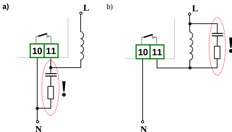
Figure 4.18. kết nối mạch triệt tiêu:
