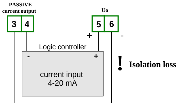
Figure 4.21. Kết nối ngõ ra dòng passive (chỉ dành cho thiết bị có ngõ ra dòng passive)
