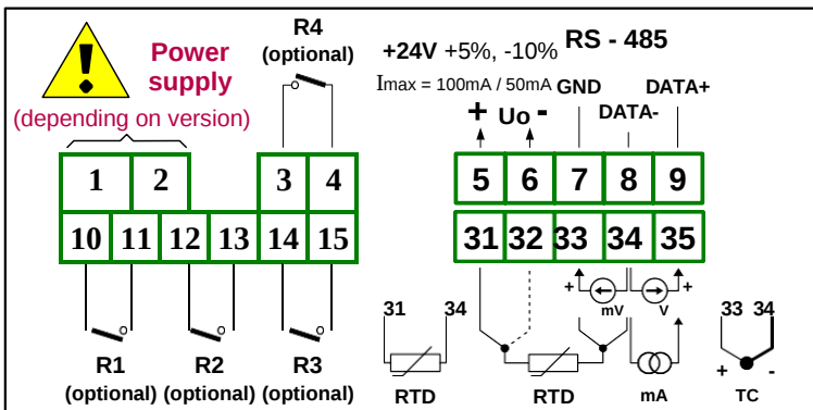
Figure 4.8. thiết bị chân kết nối (bốn ngõ ra role)
