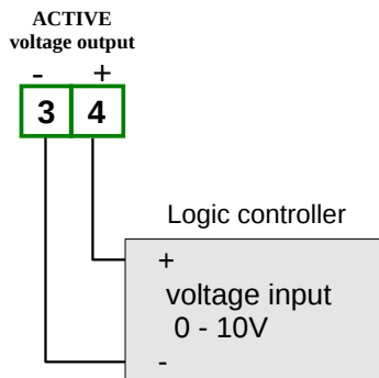
Figure 4.22. Kết nối ngõ ra điện áp active (chỉ dành cho thiết bị có ngõ ra điện áp active)
