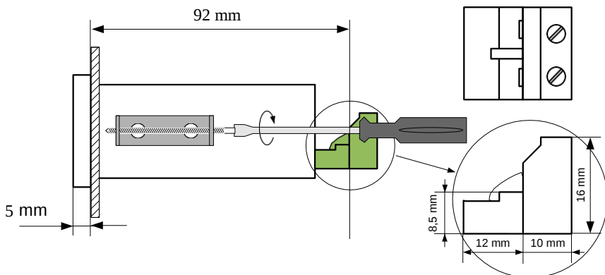
Figure 4.3. Lắp đặt giá đỡ và kích thước của đầu nối.
